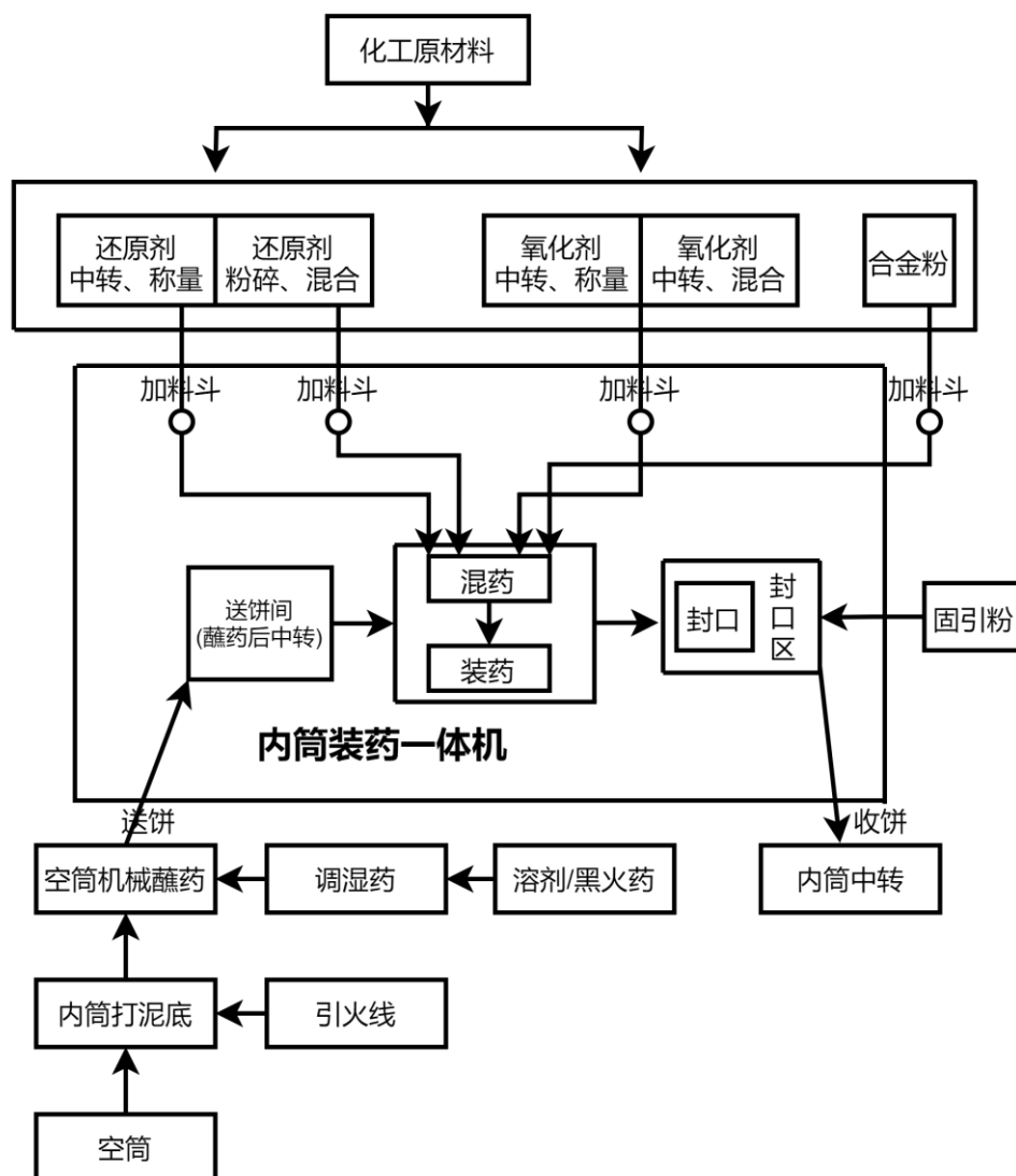
图 2-2: 内筒装药一体机组合烟花内筒效果件(不含亮珠)生产工艺流程图
