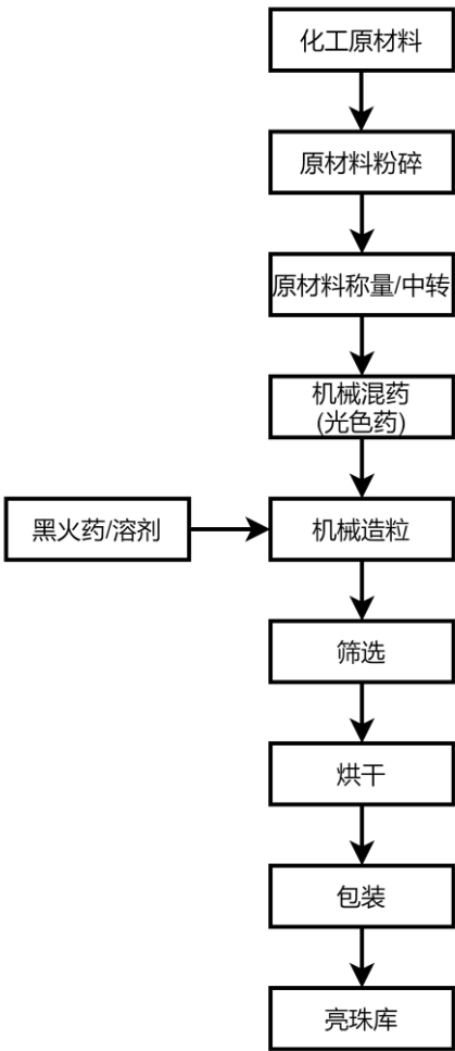
图 2-5：亮珠（仅限自产自用）生产工艺流程图
