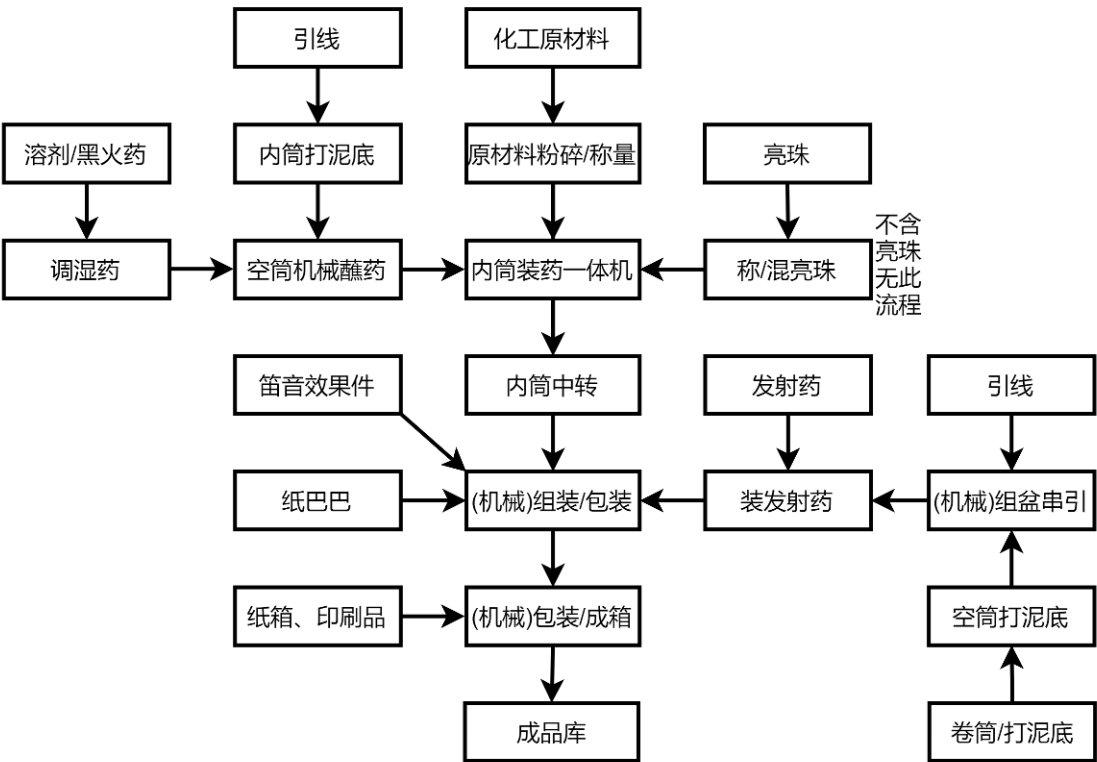
图 2-4：C 级组合烟花类生产工艺流程图
