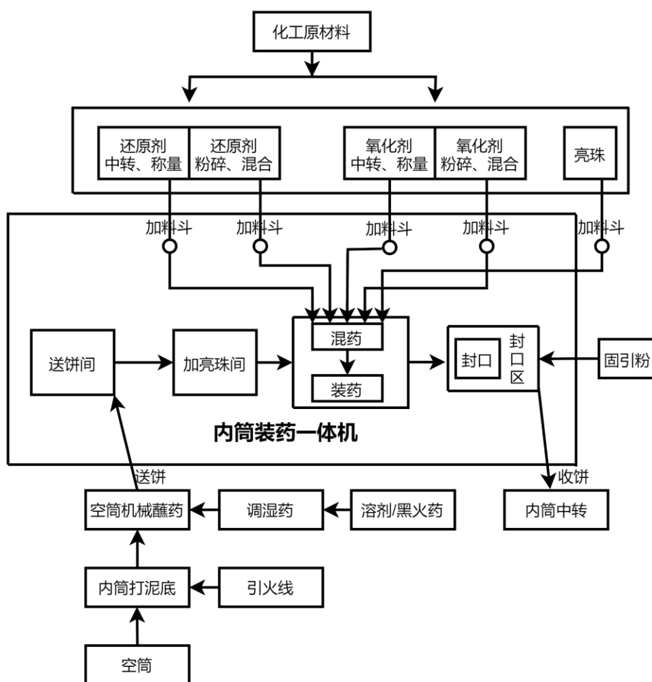
图 2-1：内筒装药一体机组合烟花内筒效果件(含亮珠)生产工艺流程图
