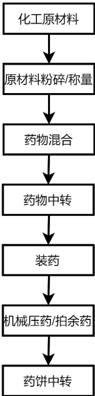
图 2-3：笛音效果件生产工艺流程图
