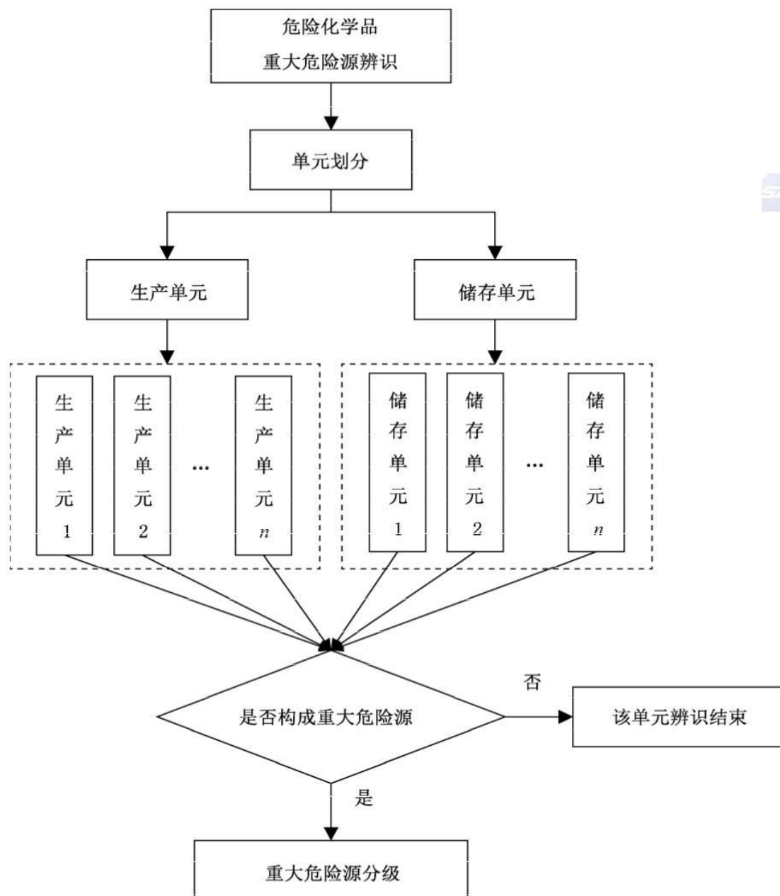
图 3.6-1 重大危险源辨识流程图
