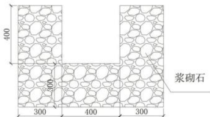
图 2-5 截水沟横断面图
