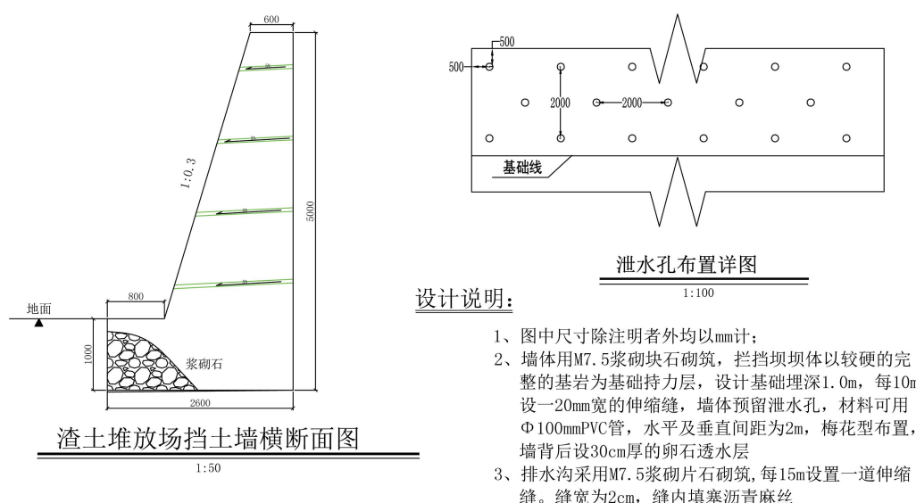
图 2-5 挡土墙设计示意图
